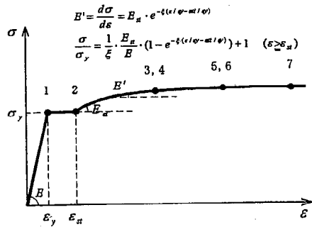
(a) 単調載荷経路 (新技術小委員会)
