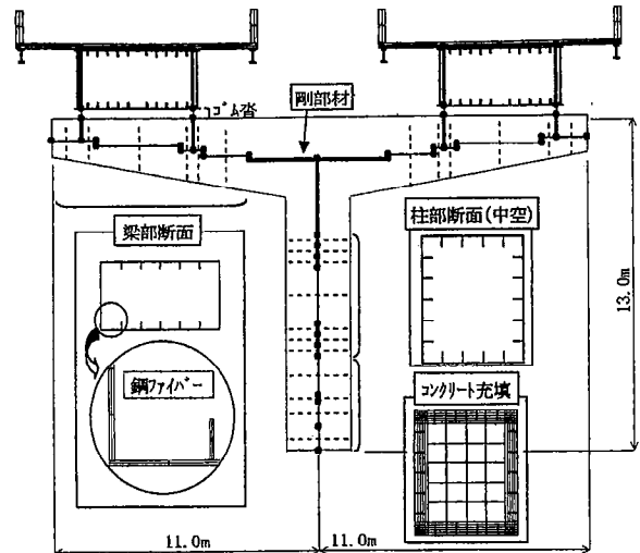
図-13 T型鋼製橋脚の解析モデル
