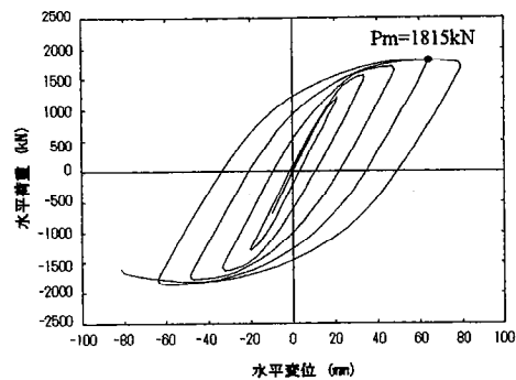
(a) 実験結果 (M20)
