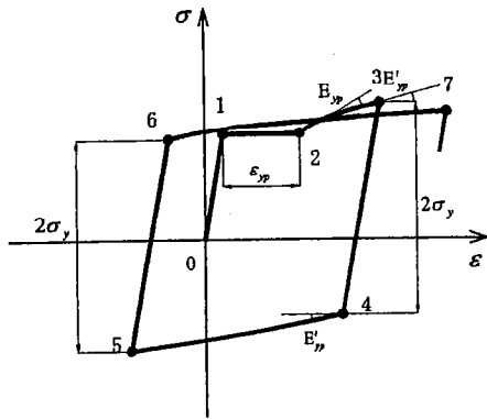
(b) 繰返し載荷経路 (新技術モデル)
