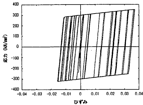
(a) 応力-ひずみ曲線 (鋼)
