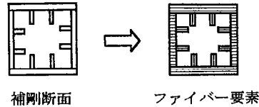
(b) ファイバー要素分割図
