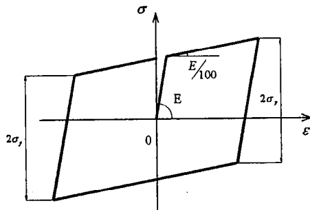
図-2 バイリニアモデル (移動硬化則)
