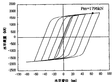
(c) 解析結果 (バイリニアモデル)
