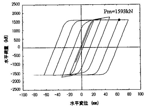
(b) 解析結果 (新技術モデル)
