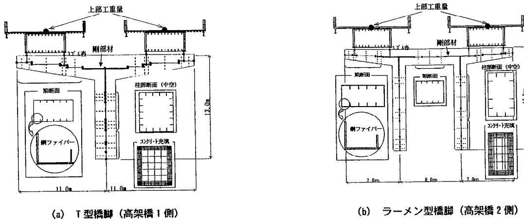
図-2 橋脚形状およびモデル化
