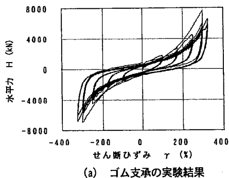
(a) ゴム支承の実験結果
