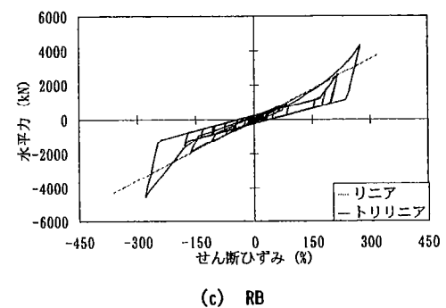
図-4 ゴム支承の応答履歴
