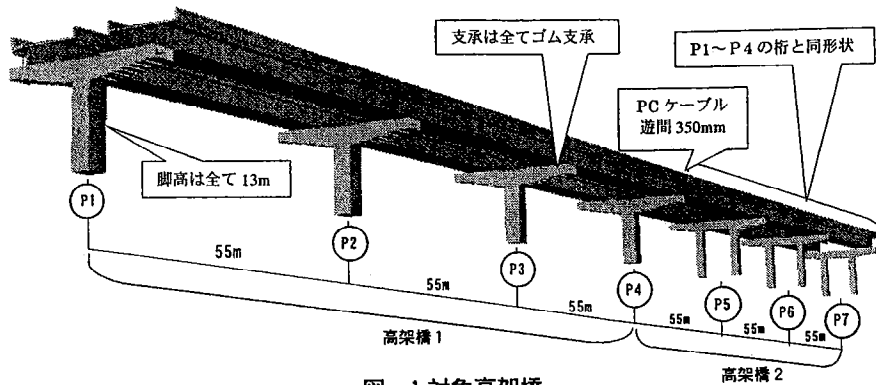
図-1 対象高架橋
