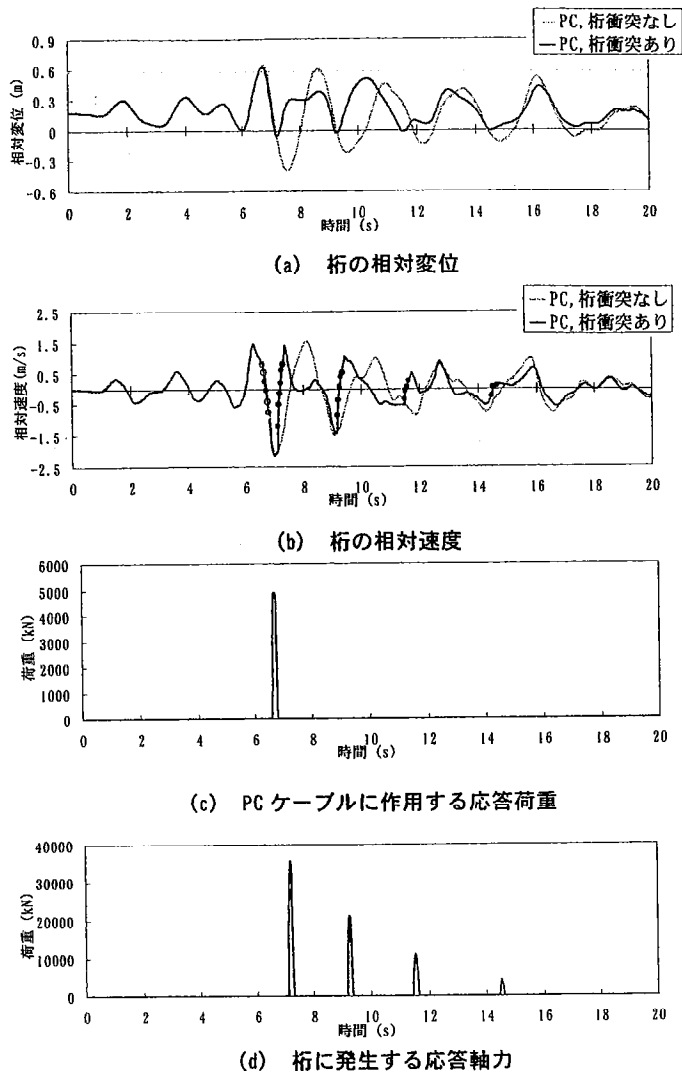
図-13 遊間175mm, 周期差1.5の応答値
