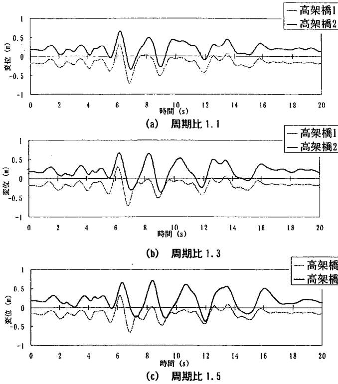
図-10 桁の応答変位
