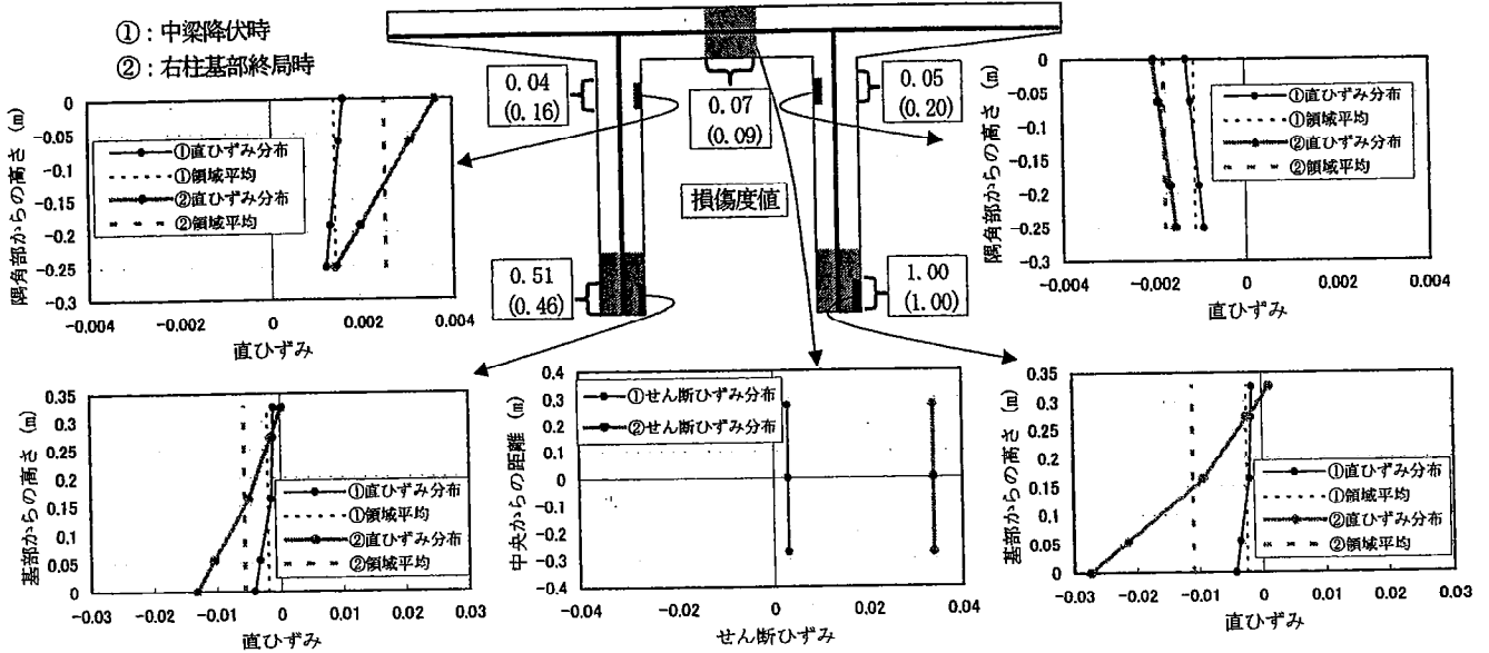
図-9 柱終局時ひずみ分布 (ケース2)
