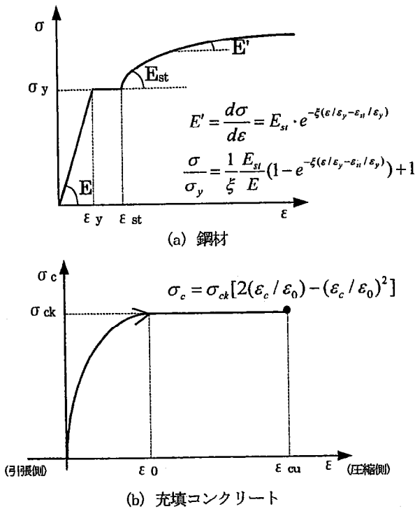
図-3 材料構成則
