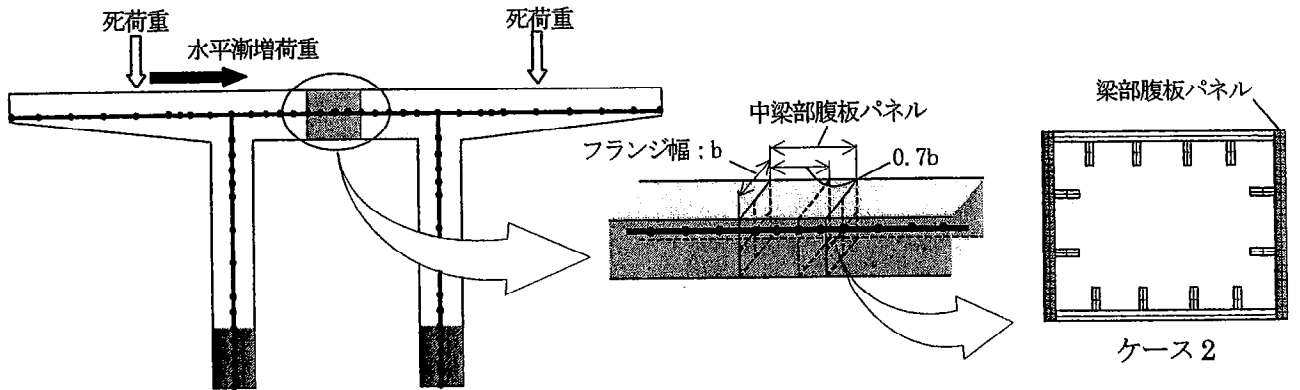
図-6 梁部せん断座屈を考慮した解析モデル
