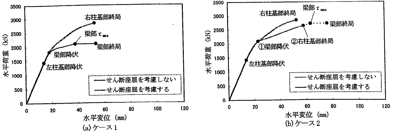
図-8 梁実験スケルトンを組み込んだ解析
