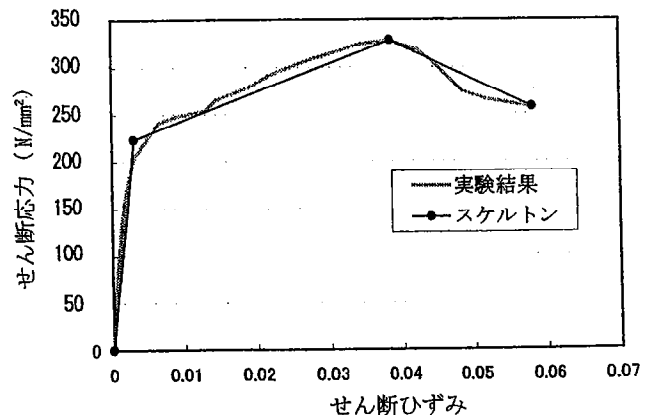
図-7 実験結果のスケルトン (ケース 2 の場合)
