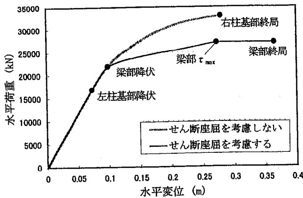
図-12 実橋脚の解析結果
