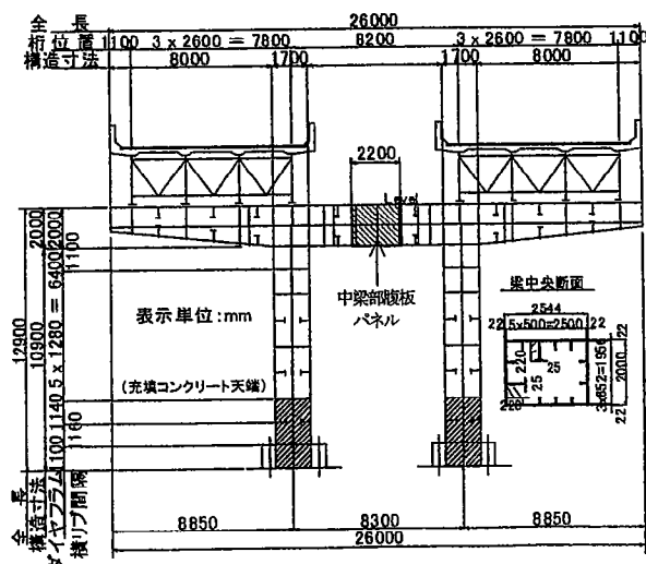
図-1 対象ラーメン橋脚
