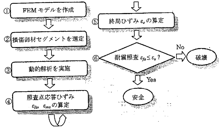
図-9 耐震照査のフロー
