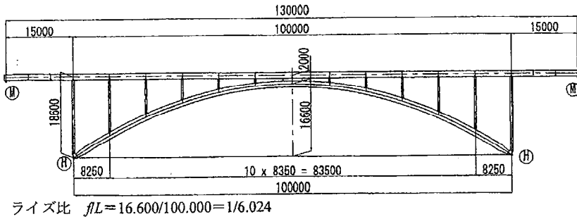
(a) 側面図
