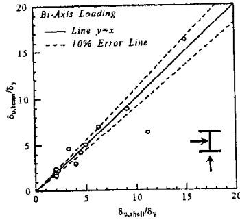
図-8 2方向載荷時の終局ひずみ算定式の検証
