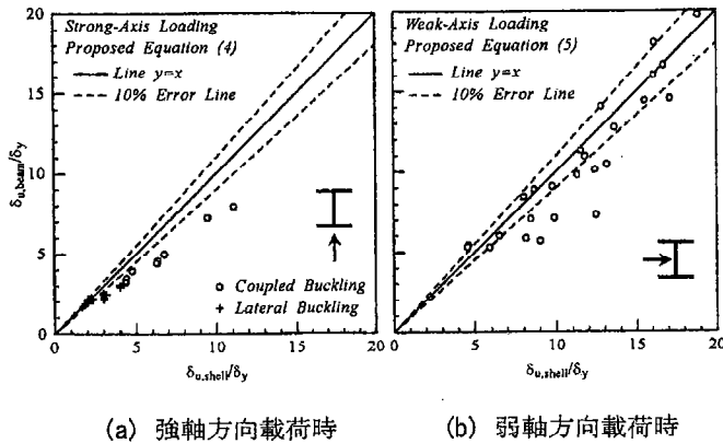
図-7 修正終局ひずみ算定式の検証
