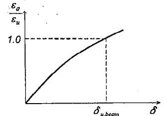
(b) はり要素の Pushover 解析
