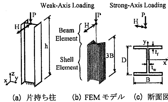
図-3 片持柱の解析モデル
