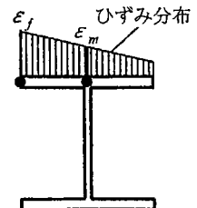
図-5 フランジにおけるひずみ照査箇所
