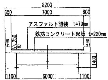
(b) 断面図
