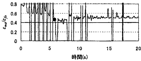
(a) \epsilon_{md}/\epsilon_{fa} の時刻歴
