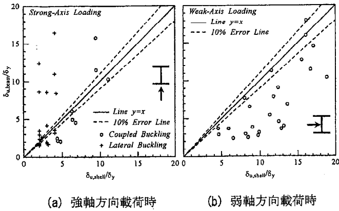
図-6 終局ひずみ算定式の検証
