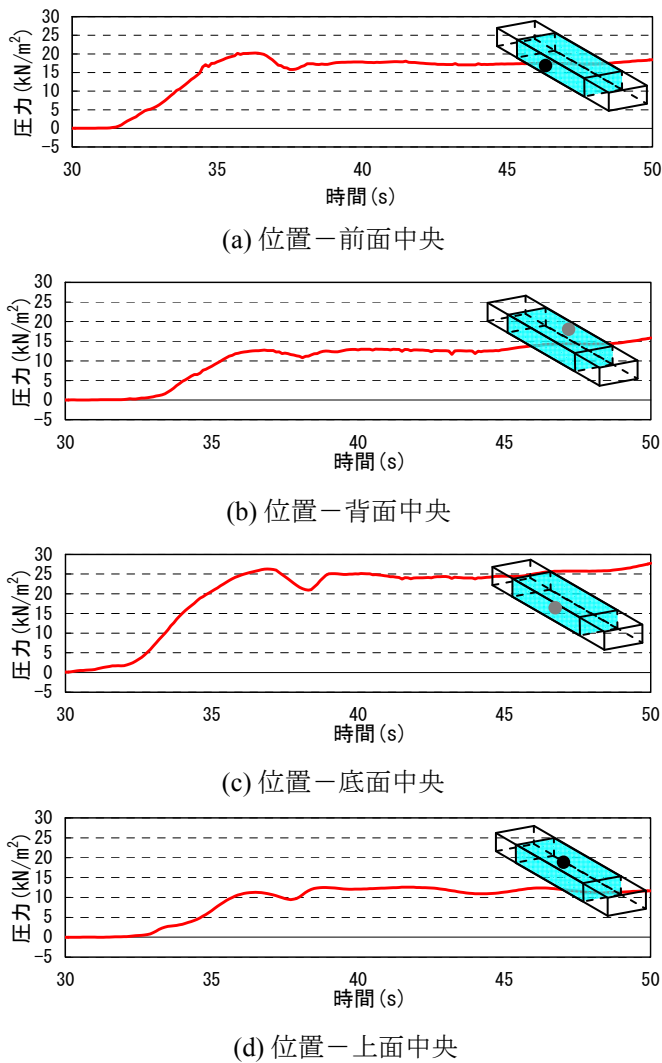
図-12 桁に作用した圧力
