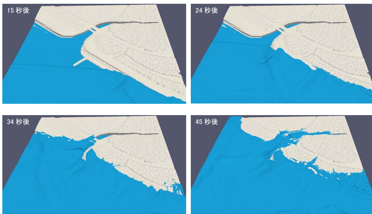
図-10 3次元津波解析結果（解析領域全体）
